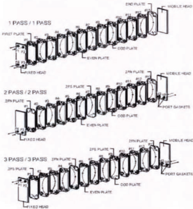
(Circulation du même côté) Figure 1.10 Arrangements de passes typiques pour tous les modèles standards
