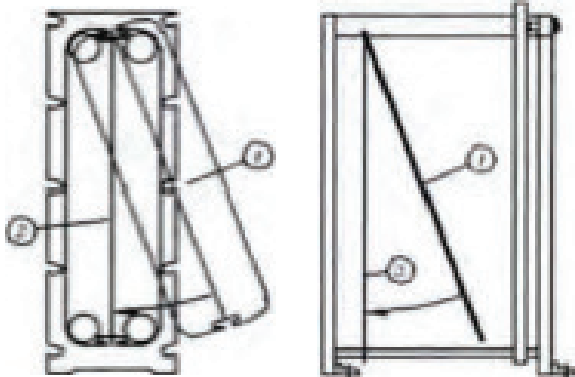
Figure 4.4 - La fixation des plaques
