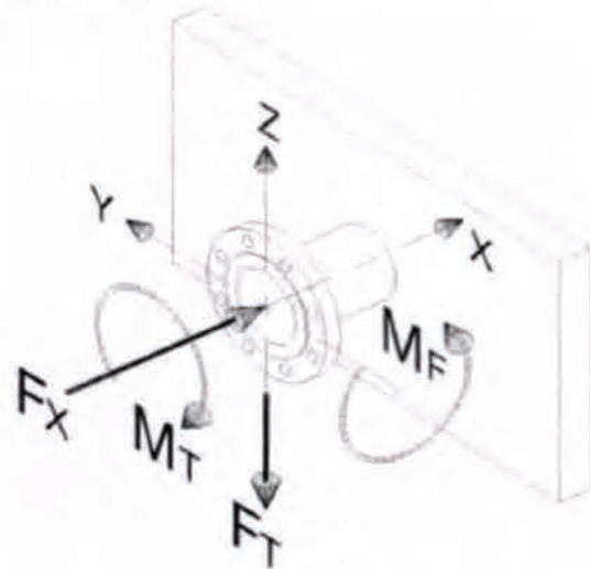
Figure 2.4 Charge de tubulure & axes de références
