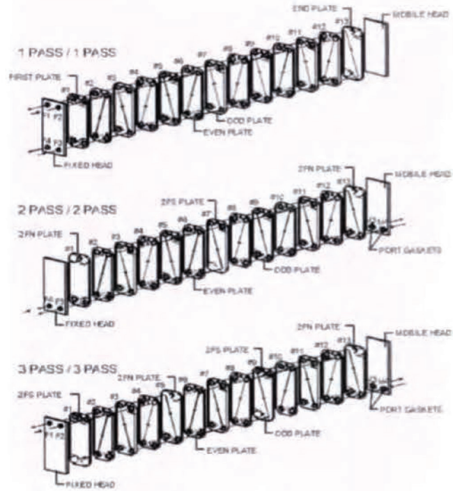
(Circulation diagonale) Figure 1.11 Arrangements de passes typiques pour tous les modèles spéciaux
